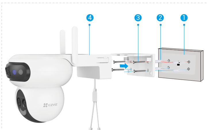
Afb. 2 Muurmontage
