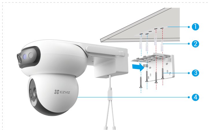
Afb. 1 Plafondmontage
